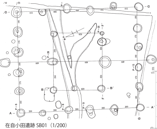
第 22 図 在自小田遺跡遺構配置図と SB01 平面図 (池ノ上他編 1994 から転載)
