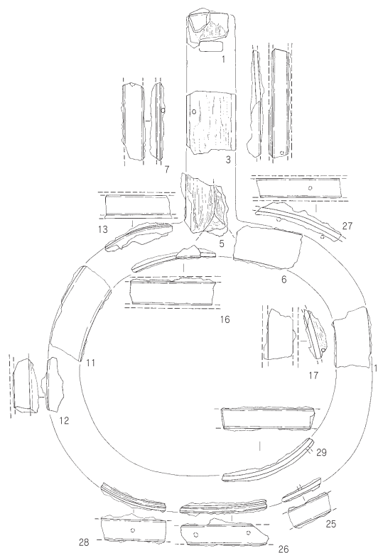
第6図 勝浦峯ノ畑古墳出土木芯鉄板張輪鏡(1/3、池ノ上他編2011から転載)
